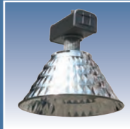
Name : Highbay Luminaire Code : 0361 - 1 Dimensions : 508 x H530(20")
